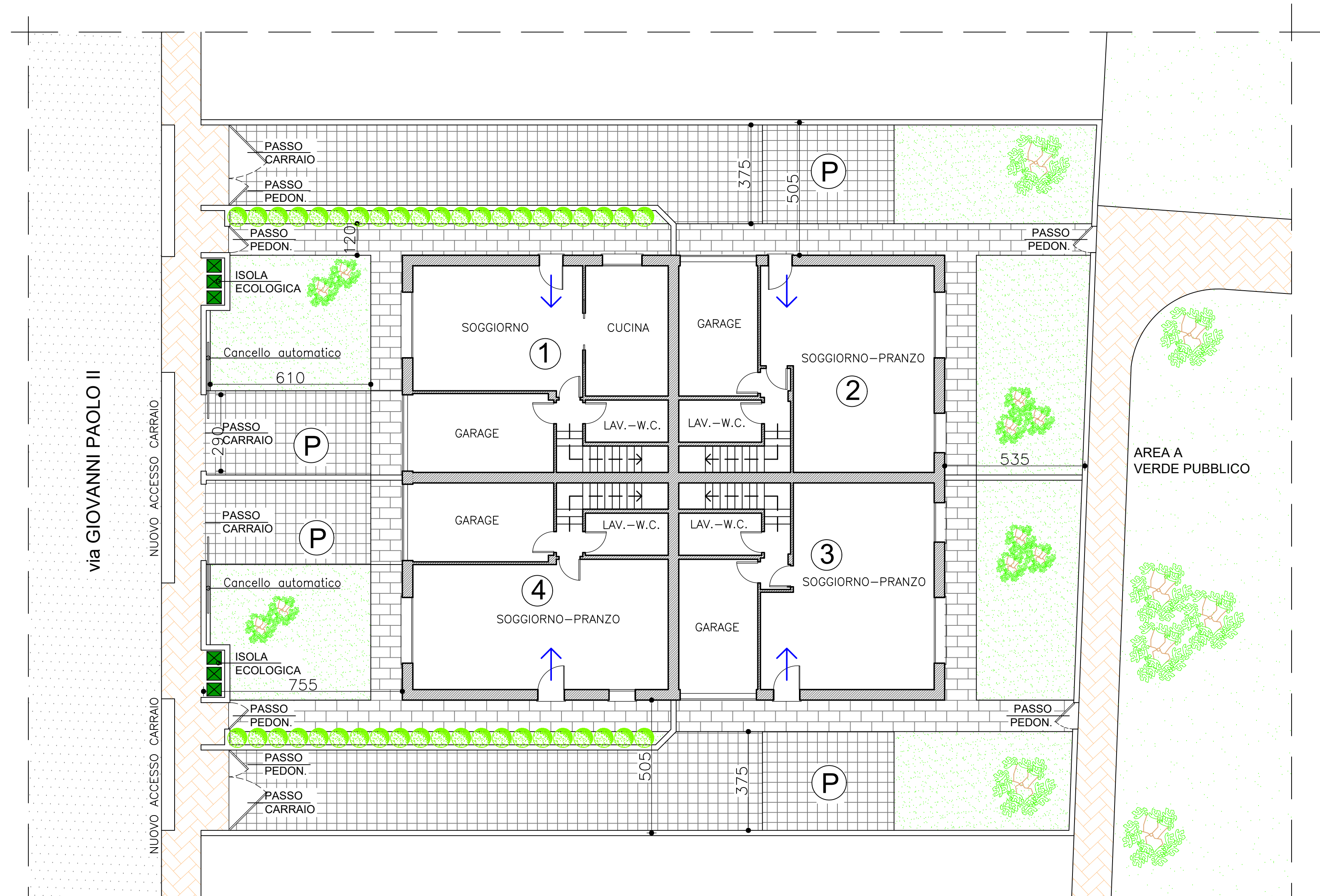
SISTEMAZIONE ESTERNA scala 1:200
